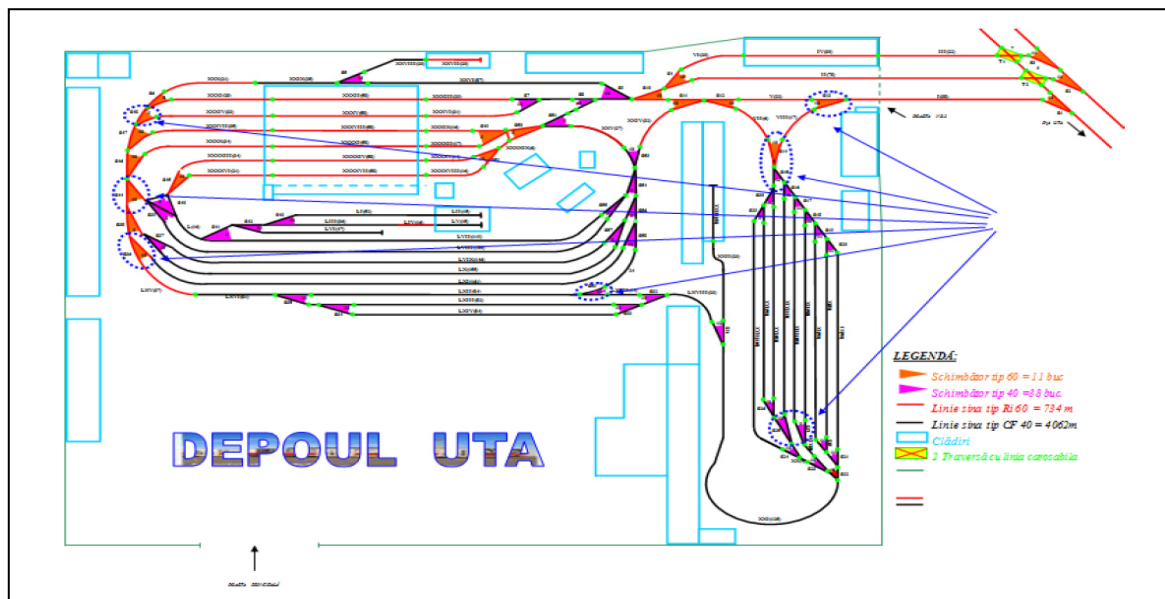
Planul general al depoului UTA
